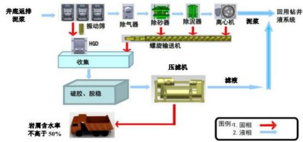
图 2-7 泥浆循环系统工艺流程简图
