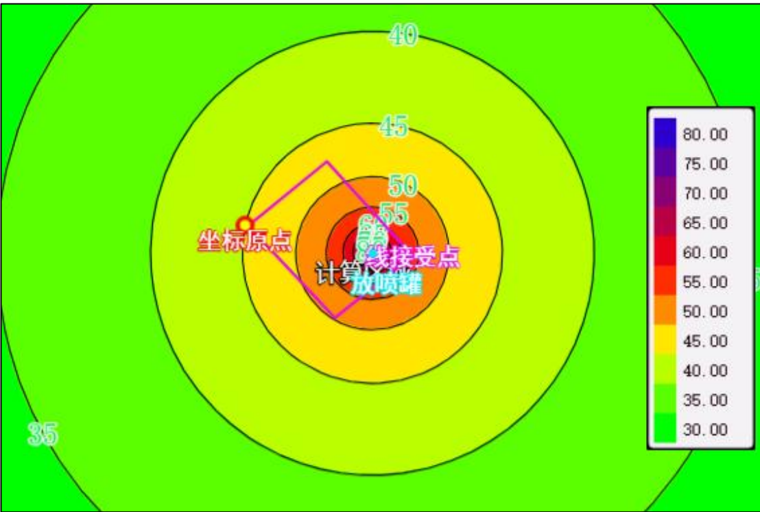
图 4-2 放喷期间噪声等声线图
