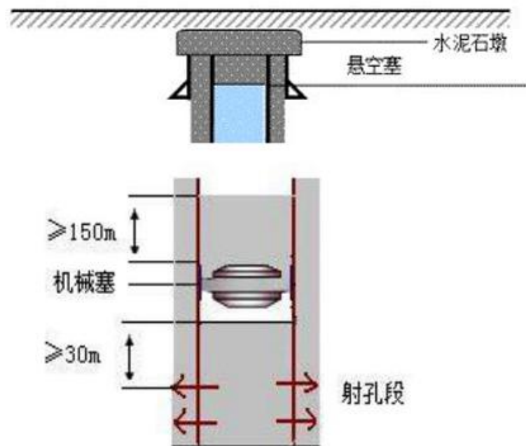
图 2-5 井口及射孔封堵示意图
