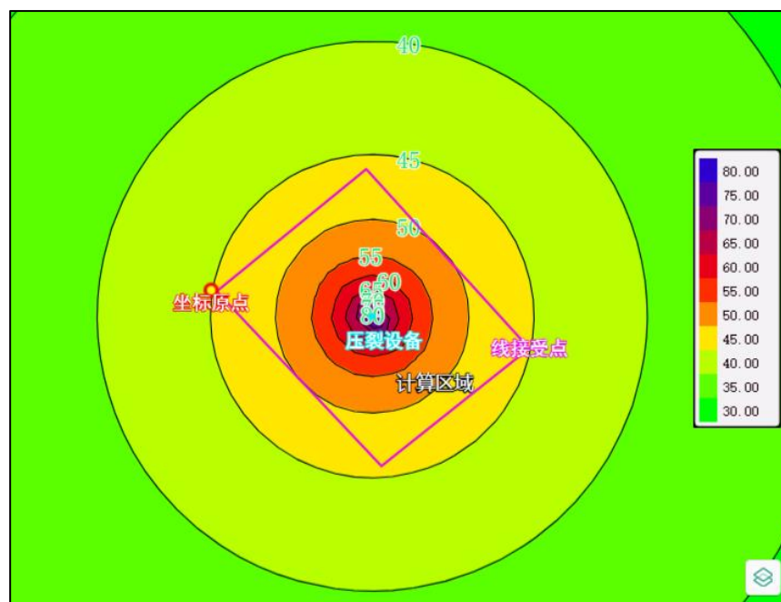
图 4-1 压裂期间噪声等声线图
