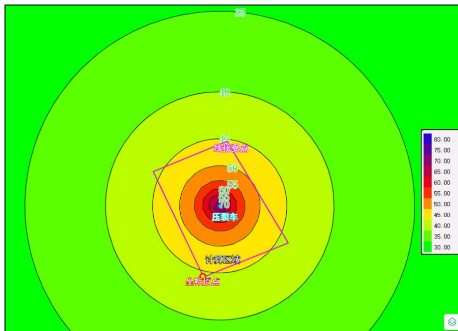
图 4-1 压裂期间噪声等声线图
