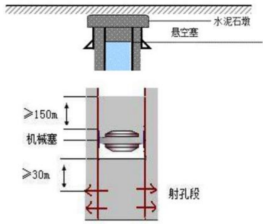
图 2-6 井口及射孔封堵示意图
