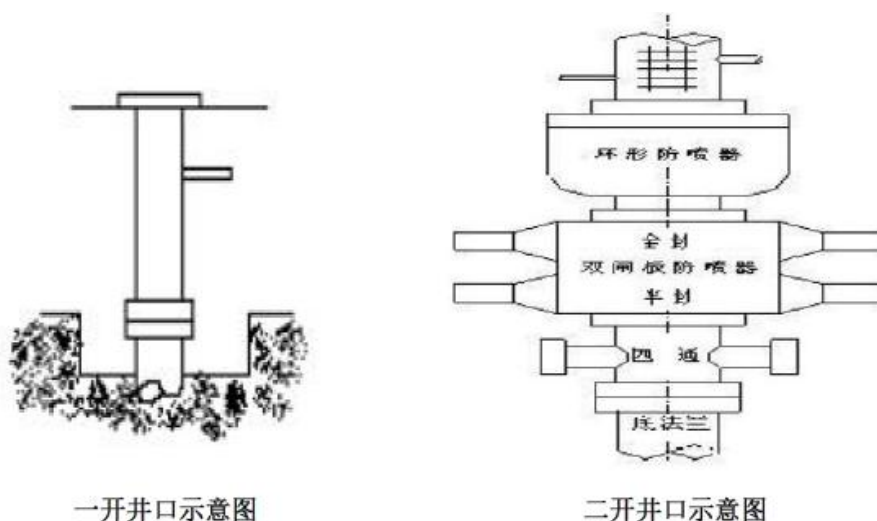
图 2-5 一开、二开井口示意图
