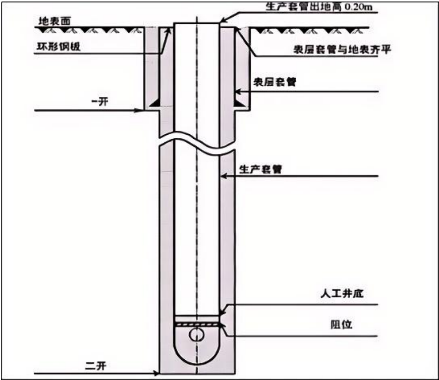
图 2-1 井身结构图
