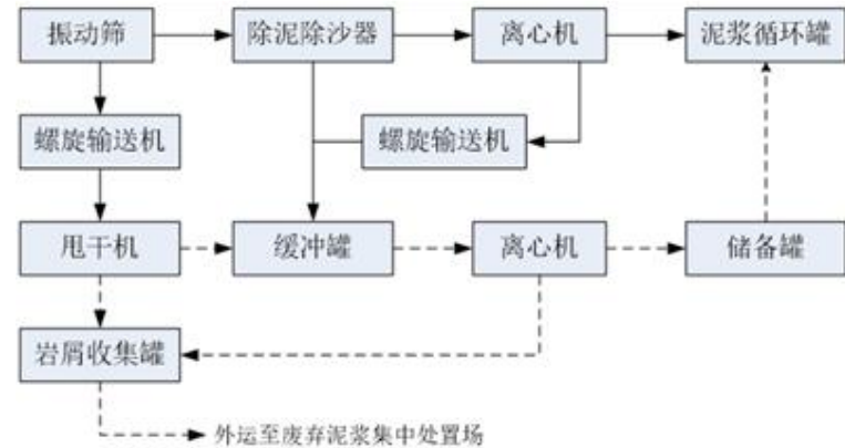
图 5-5 泥浆循环利用工艺流程图
