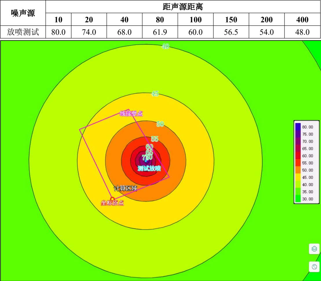
图 4-2 放喷噪声等声线图
