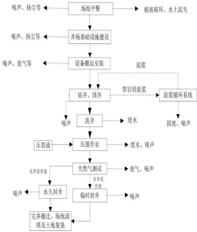
图 2-4 项目主要工艺流程及产污环节图
